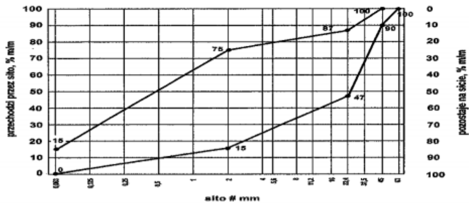
Rys. 20. Mieszanka niezwiązana 0/45 do nawierzchni z kruszywa niezwiązanego
