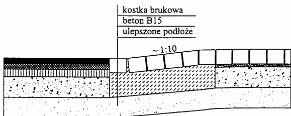
a) bez pogrubienia podbudowy (z dostosowaniem jej do kształtu progę)
