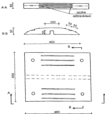
Rys. 3. Próg typu listowego długości 900 mm i wysokości 50 mm
