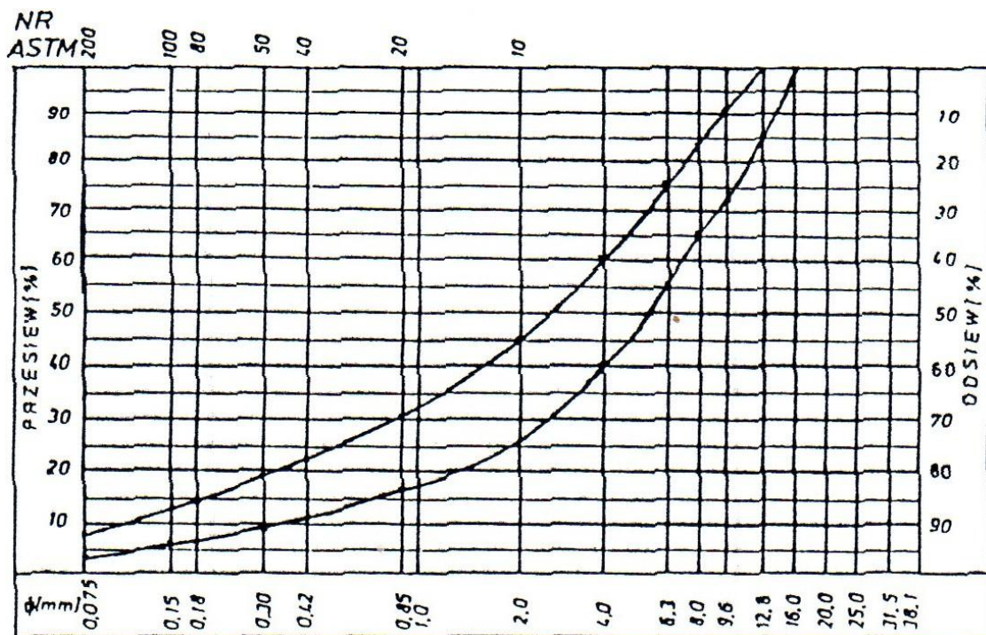
rys. 4. Krzywe graniczne uziarnienia mieszanki mineralnej 0÷16 mm do podbudowy z betonu asfaltowe
