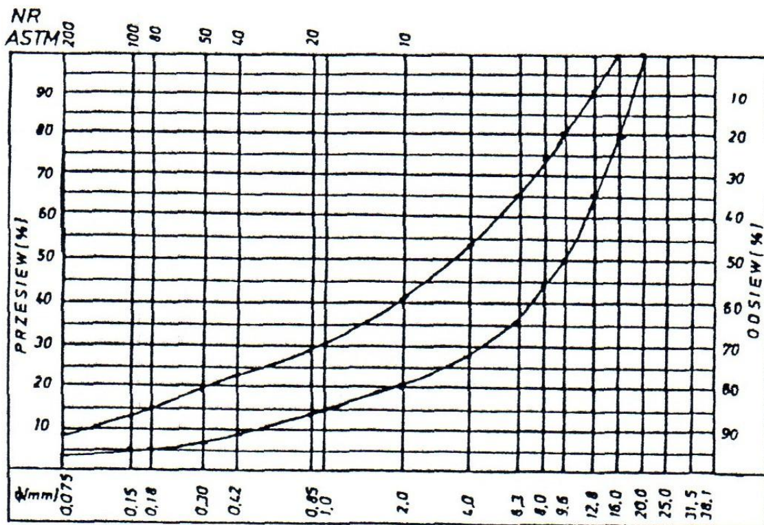
rys. 3. Krzywe graniczne uziarnienia mieszanki mineralnej 0÷20 mm do podbudowy z betonu asfaltowego dla KR 1-2
