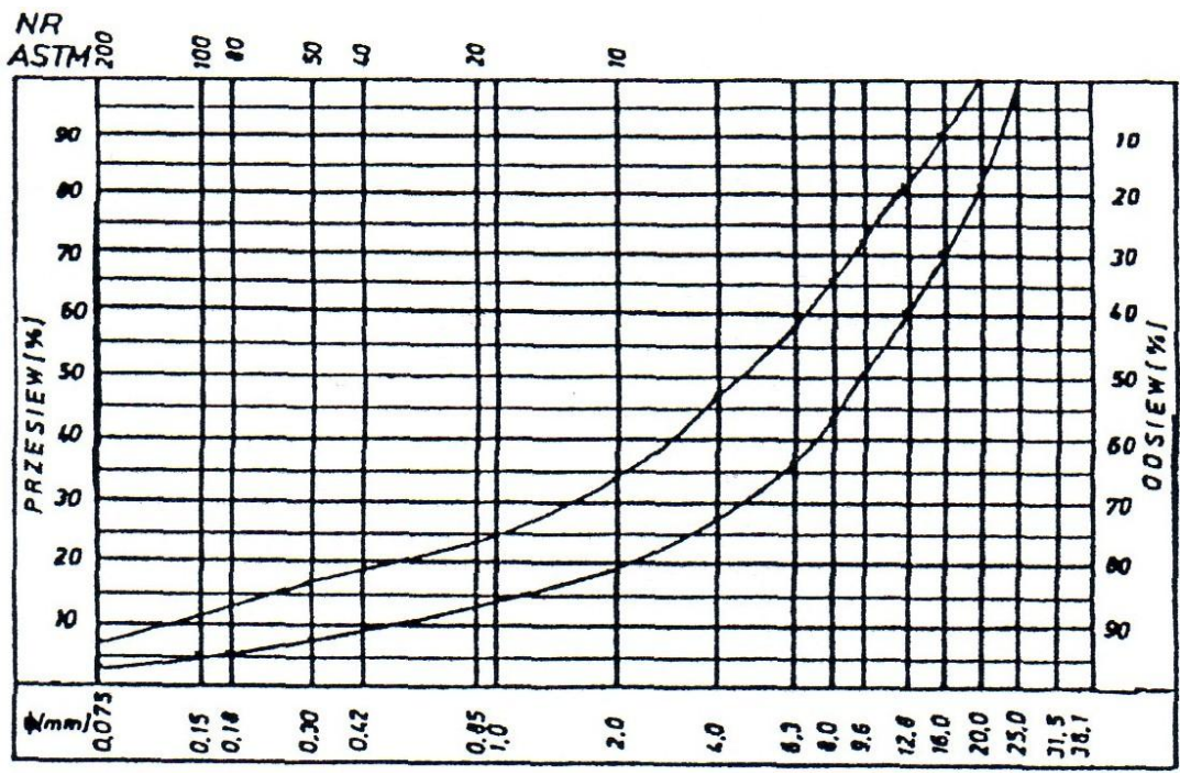
Rys. 7. Krzywe graniczne uziarnienia mieszanki mineralnej CN-25 mm do podbudowy z betonu asfaltowego dla KR 3-6.
