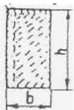
Rys. 1. Wymiarowanie krawężników
