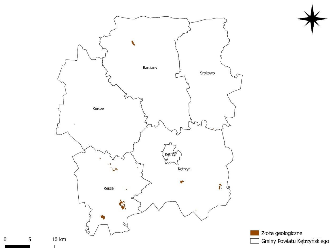
Rycina 15. Złoża kopalin na terenie Powiatu Kętrzyńskiego (wg stanu na dzień 31.12.2020 r.)
