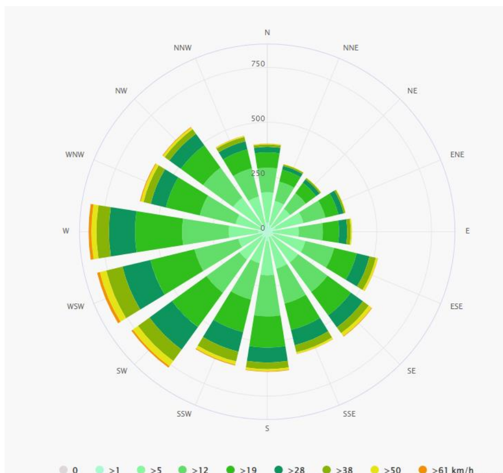
Rycina 5. Róża wiatrów dla Miasta Kętrzyn
