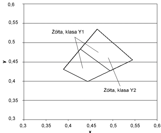
Rys.2. Współrzędne chromatycyjnosc x,y dla barwy zoltej oznakowania
